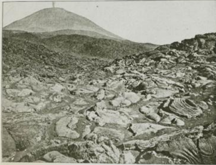
Cóno de ceniza del Vesubio y arroyo de lava. En la superficie se ve lava en forma de "flawn".
